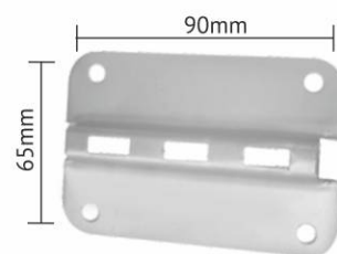
SINGLE SHELF MINI CHANNEL DC-06
