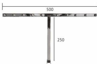
'T' TYPE HANGER STAND DC-139
